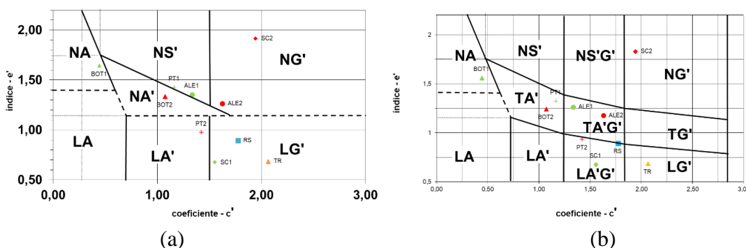
Figura 2: Ábacos para classificação segundo metodologia MCT.
