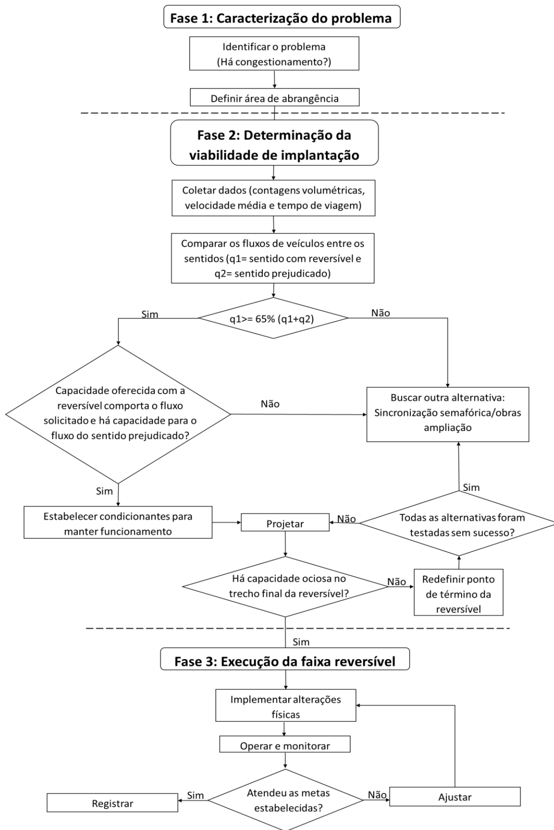
Figura 2: Protocolo proposto para implantação de faixa reversível
