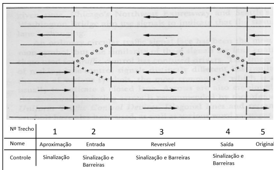
Figura 1: Configuração geral das operações de pistas reversíveis Fonte: Adaptado de Lathrop (1972)
