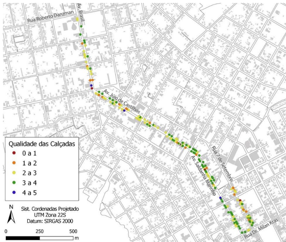
Figura 6: Índice de qualidade da infraestrutura das calçadas no cenário de estudo
