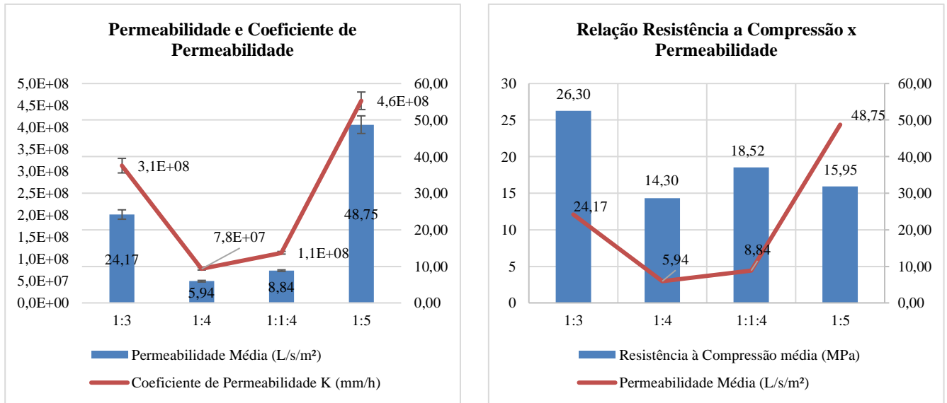
(a) Gráfico – Permeabilidade e Coeficiente de Permeabilidade (b) Gráfico –Relação entre Resistência e Permeabilidade. Figura 7: Gráficos de Permeabilidade
