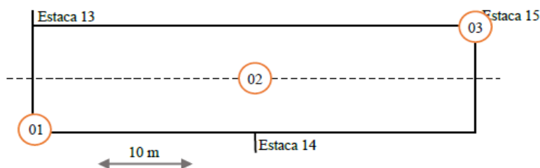
Figura 3: Esquema de aplicação do SSG no trecho experimental avaliado pela UFC
