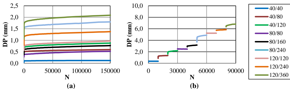
Figura 5: Exemplos de curvas resultantes de solos ensaiados em (a) estágio único e (b) multiestágios no TCR
