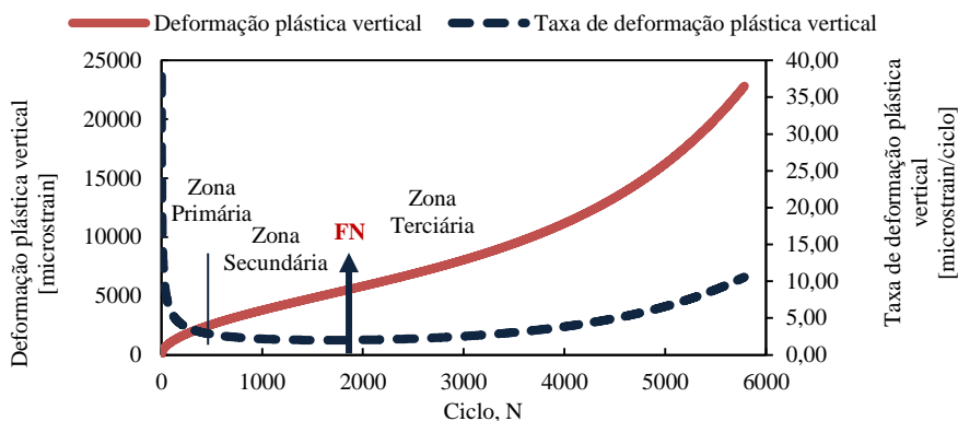
Figura 2: Relação entre a deformação total acumulada, a taxa em que as deformações ocorrem e o número de ciclos
