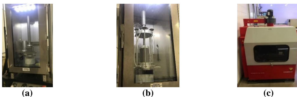
Figura 1: Equipamentos para avaliação de deformação permanente de misturas asfálticas: (a) ensaio uniaxial de carga repetida, (b) ensaio triaxial de varredura de tensões e ensaio stress sweep rutting , e (c) simuladores de laboratório
