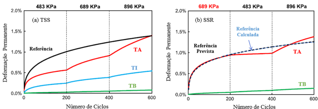
Figura 3: Comparação das curvas de ensaio do TSS e do SSR (adaptado de Kim e Kim, 2017)
